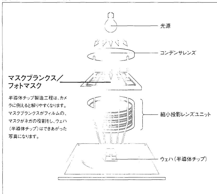
露光工程における回路パターン転写のイメージ
