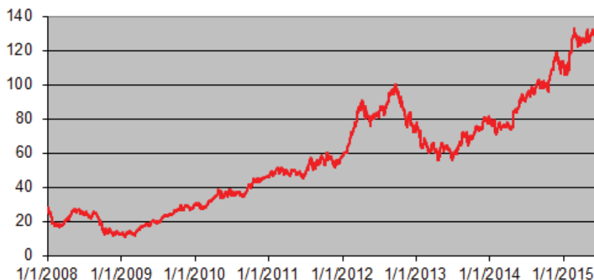
AAPL
