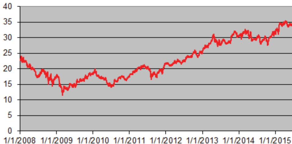
PFE
